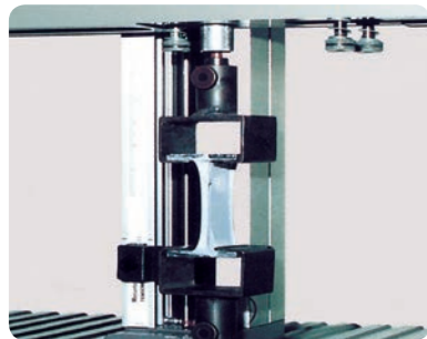
인장점착강도시험
